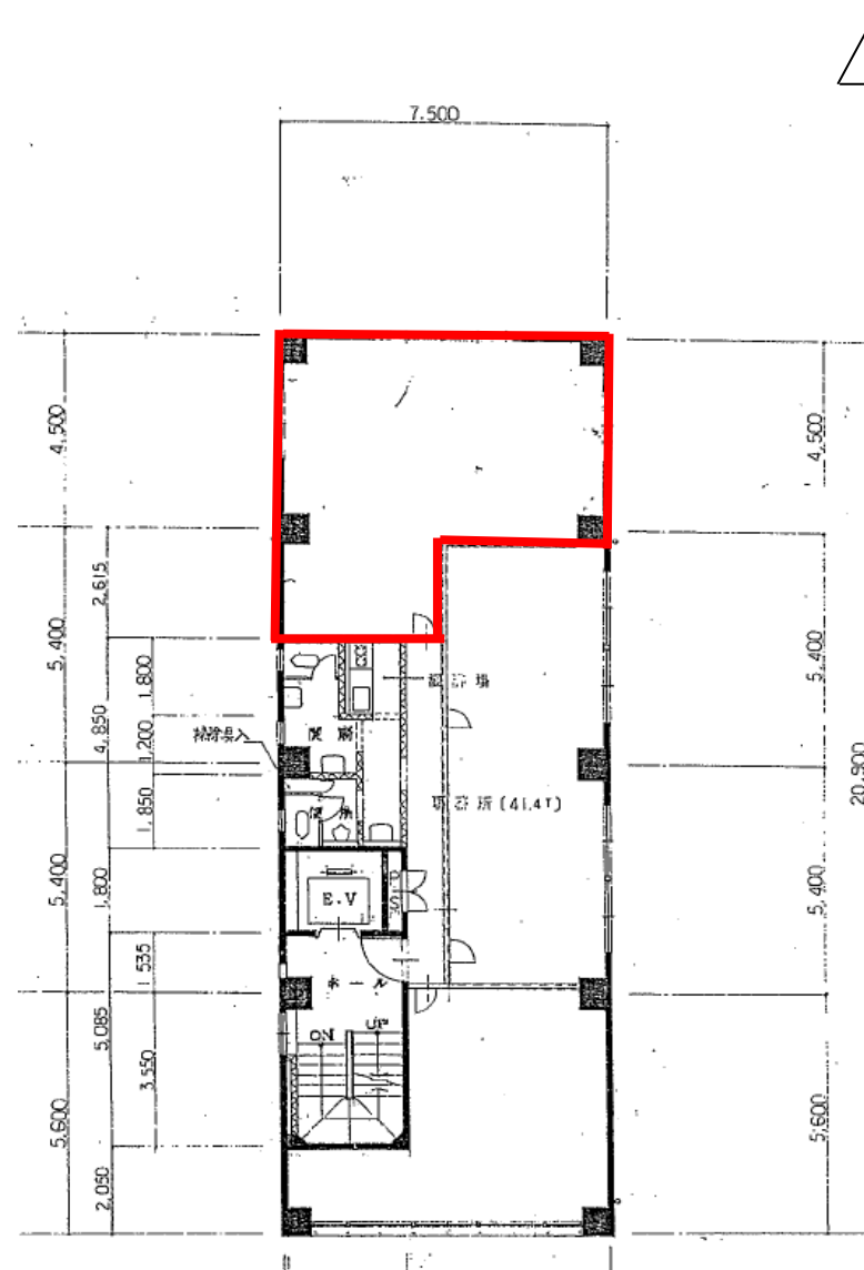
【2階平面図】
