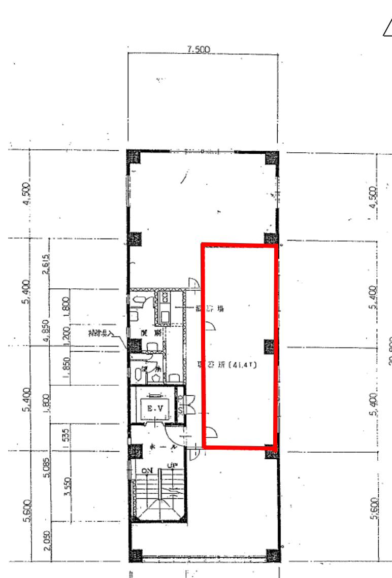
【4階平面図】
