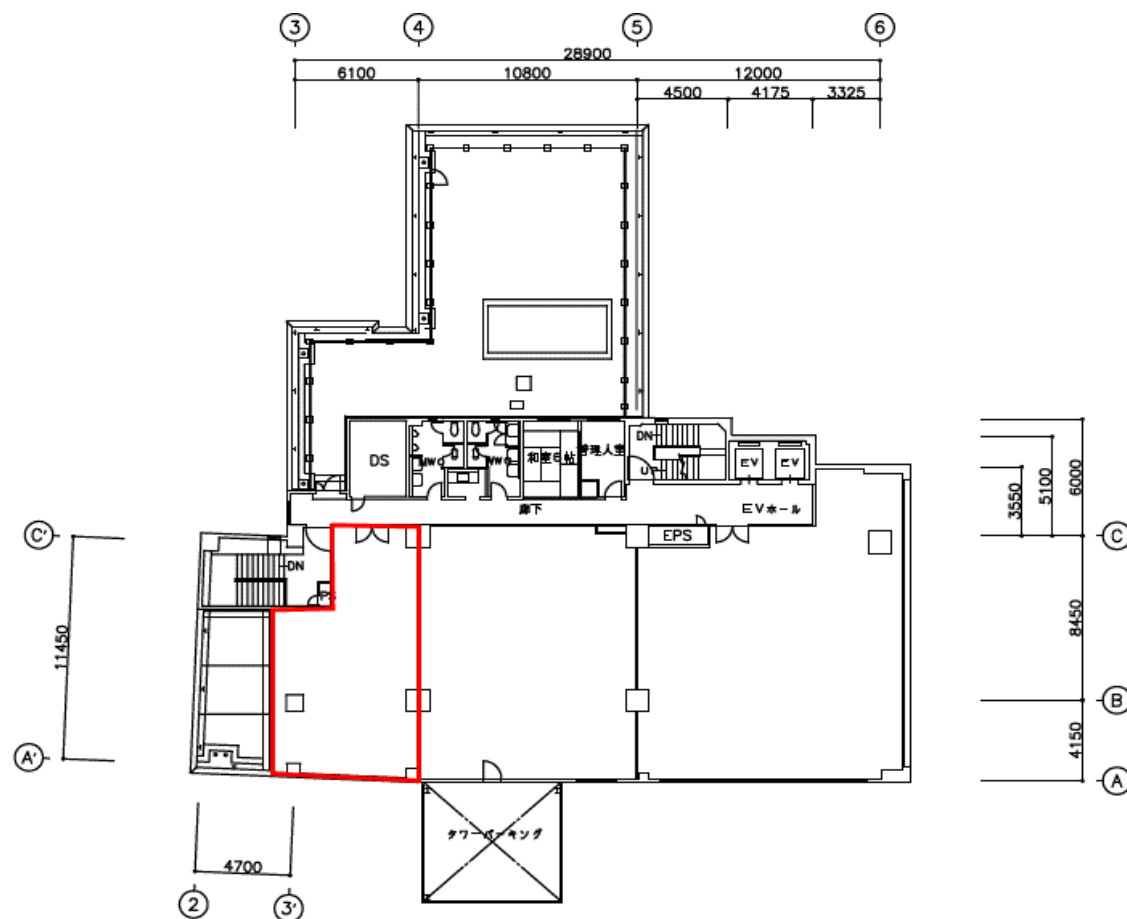
【 6F 平面図 】
